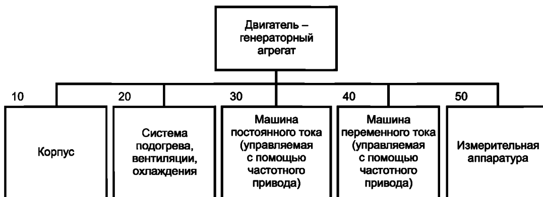
Рисунок В.2 — Диаграмма подсистем двигателя—генератора
