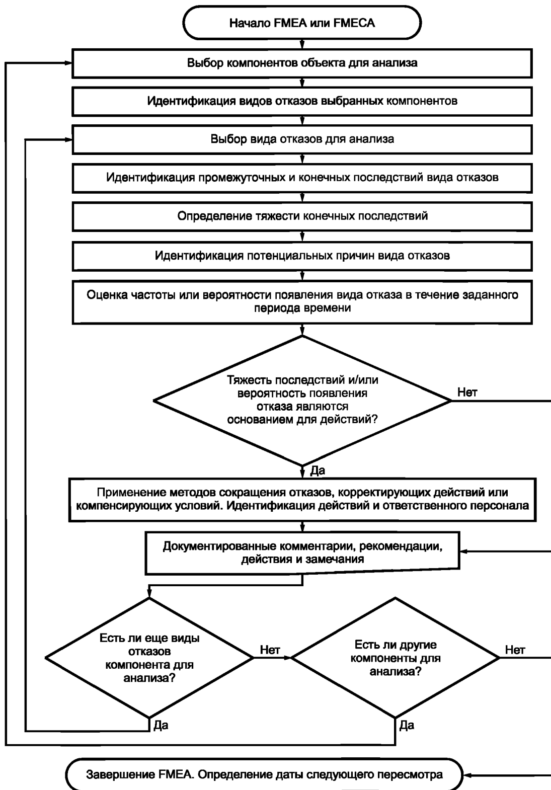
Рисунок 2 — Блок-схема анализа
