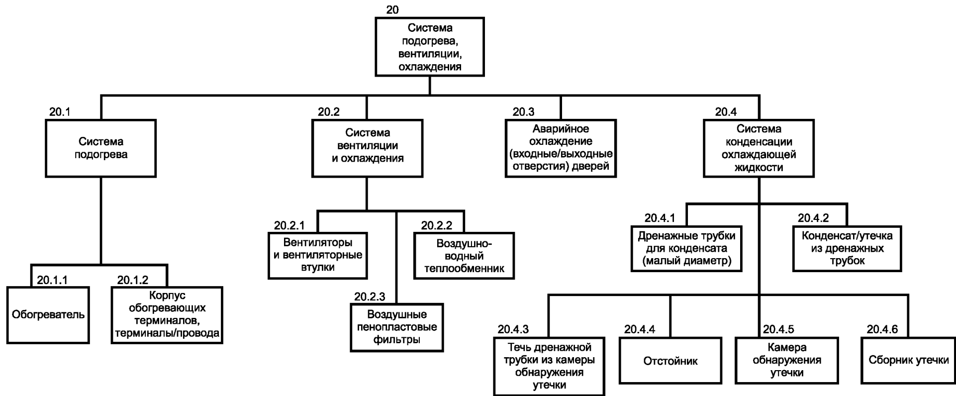
Рисунок В.3 — Диаграмма системы нагревания, вентиляции, охлаждения
