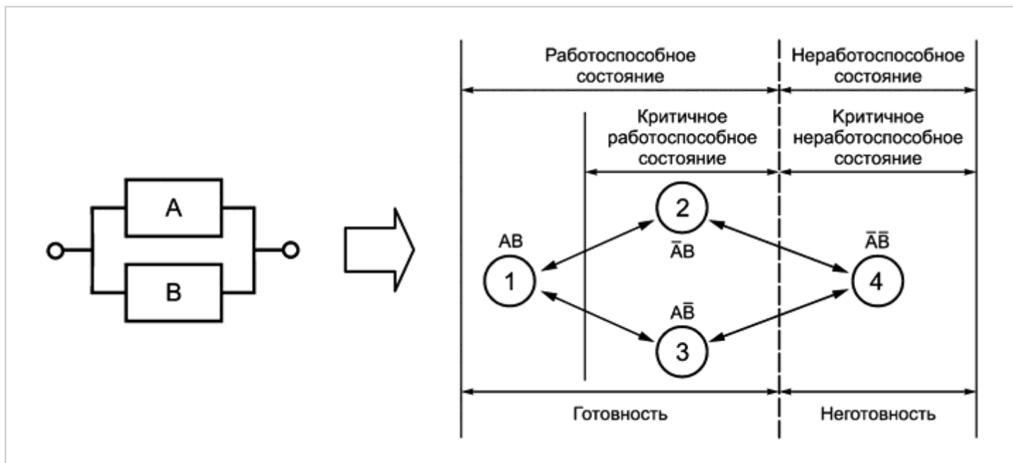
Рисунок 14 - Диаграмма состояний для простой системы с нагруженным резервом
