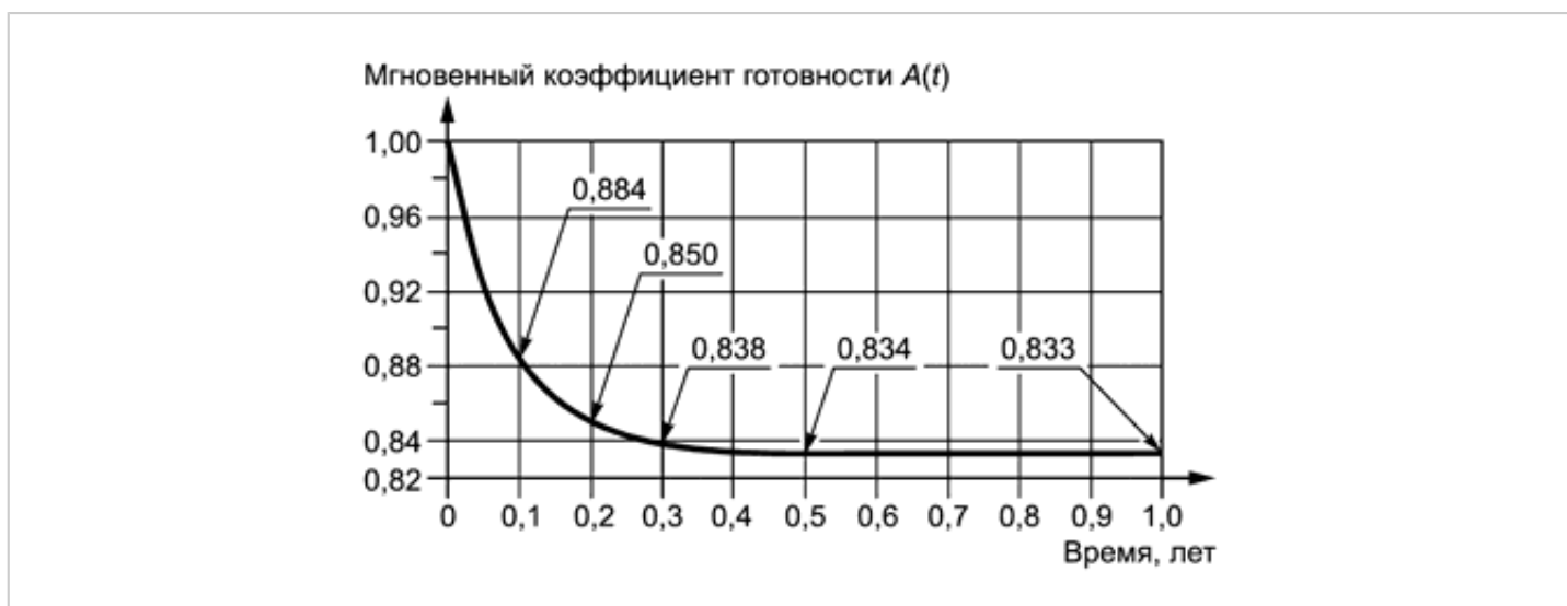
Рисунок 40 - График зависимости от времени мгновенного коэффициента готовности A(t)
