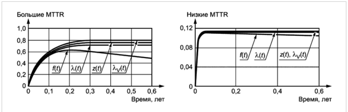
Рисунок 30 - Графики зависимости от времени z(t) и f(t)
