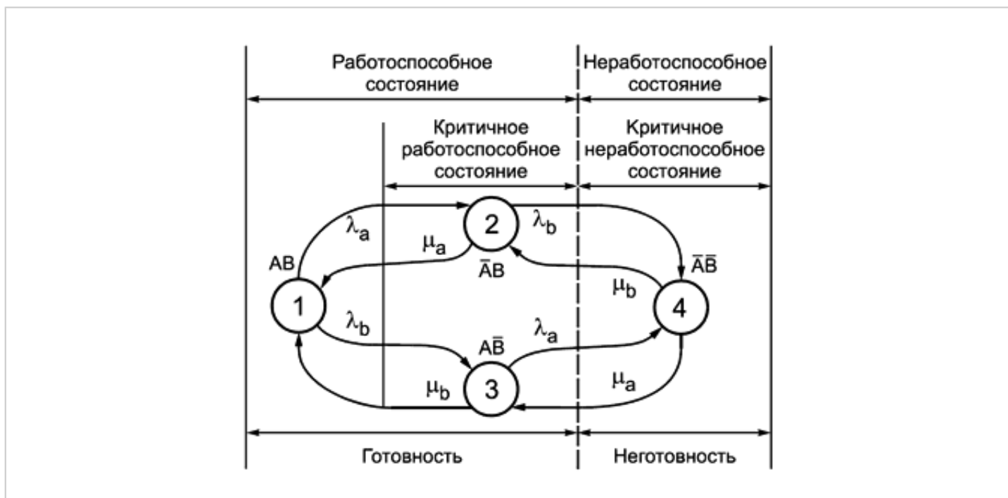
Рисунок 15 - Марковская диаграмма для простой системы с нагруженным резервом
