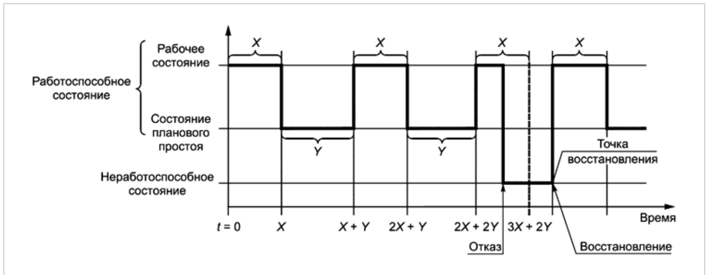
Рисунок 45 - Пример состояний элемента
