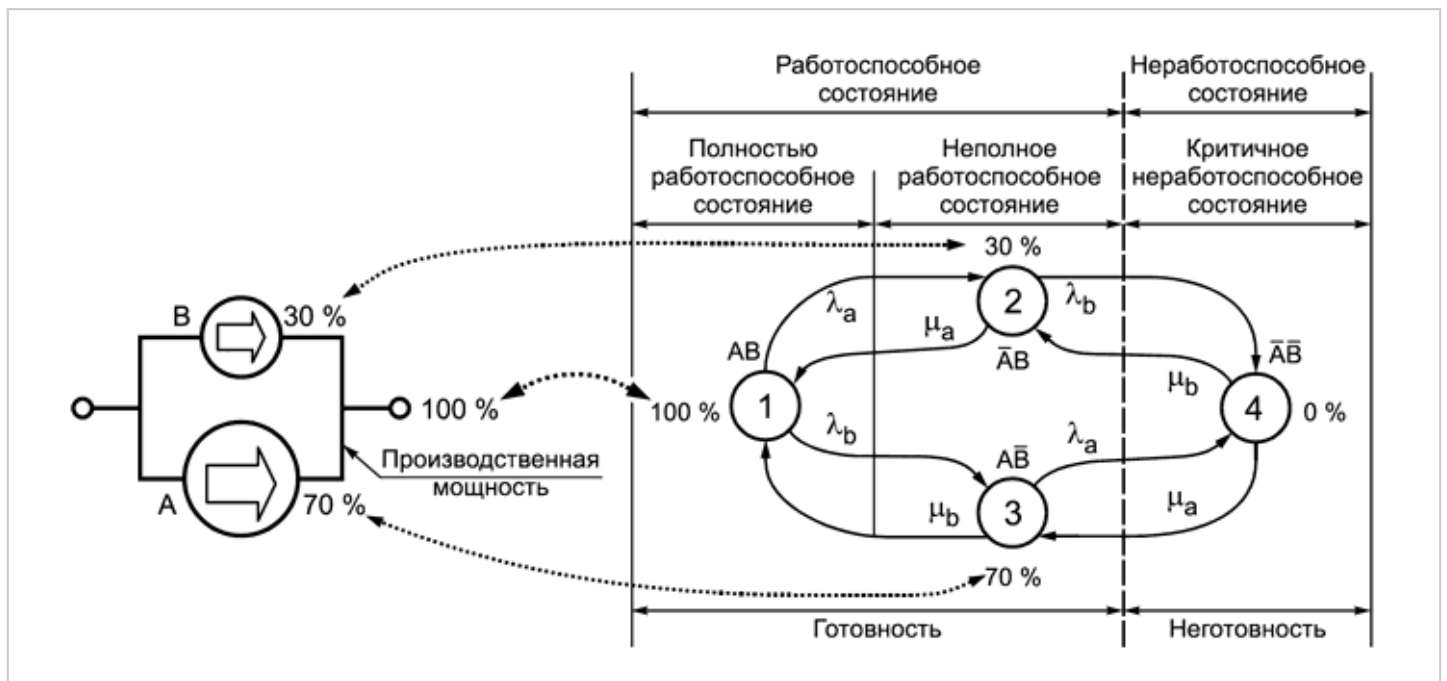
Рисунок 20 - Пример простой производственной системы
