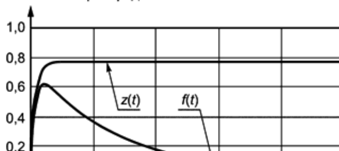
Безусловный параметр потока отказов и плотность распределения
