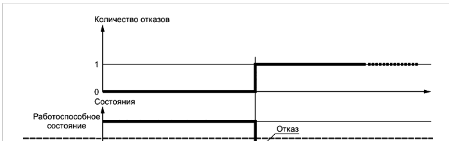
Рисунок 6 - Диаграмма состояний невосстанавливаемого элемента
