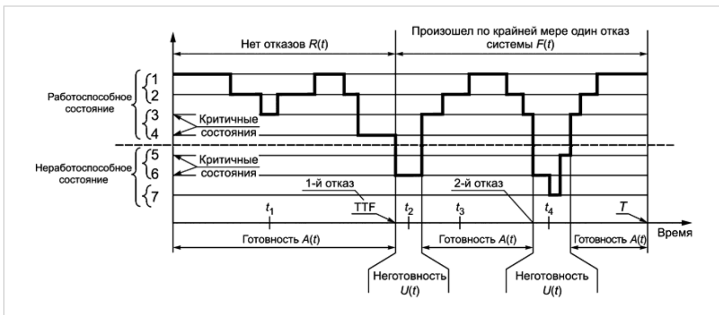
Рисунок 5 - Хронограмма, соответствующая системе, представленной на рисунке 4
