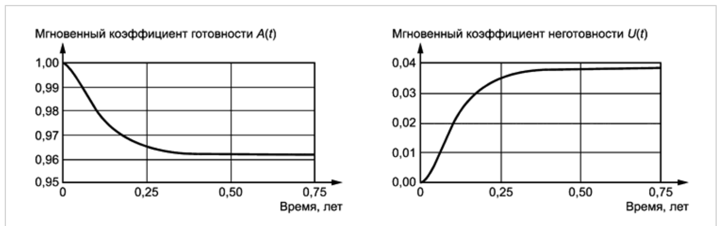
Рисунок 17 - График зависимости от времени A(t) и U(t) для марковской модели,
