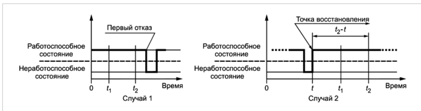
Рисунок 34 - Пример вероятности безотказной работы за период времени [t_1, t_2] для ненулевого времени восстановления элемента
