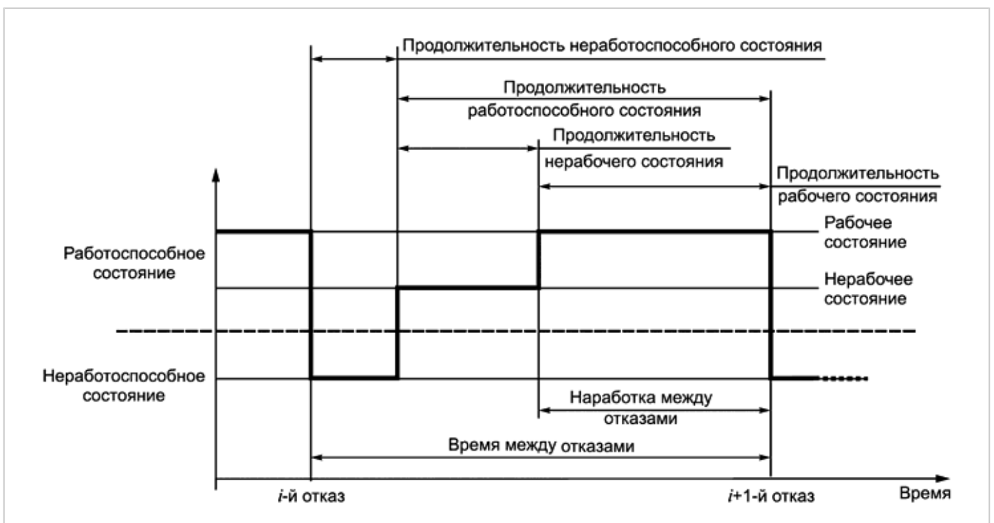
Рисунок 28 - Время между отказами и наработка между отказами
