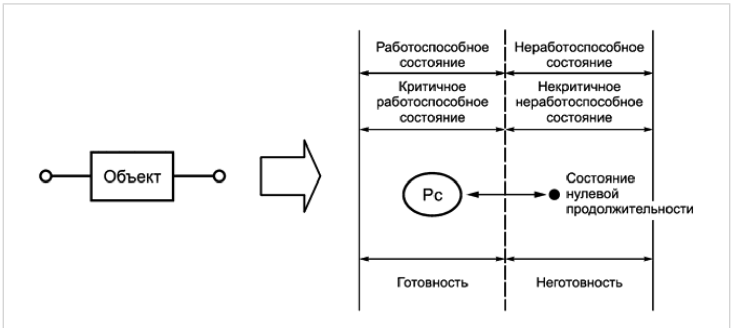
Рисунок 10 - Диаграмма состояний восстанавливаемого элемента
