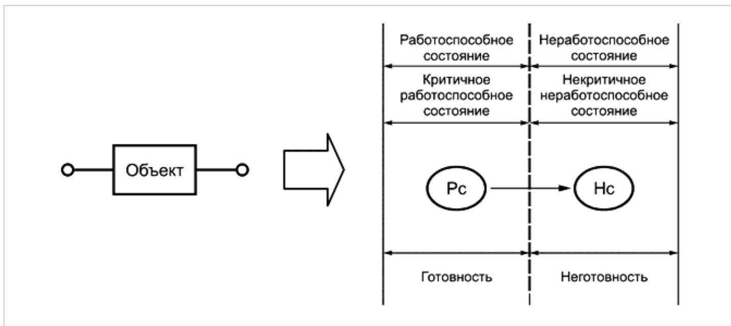
Рисунок 6 - Диаграмма состояний невосстанавливаемого элемента
