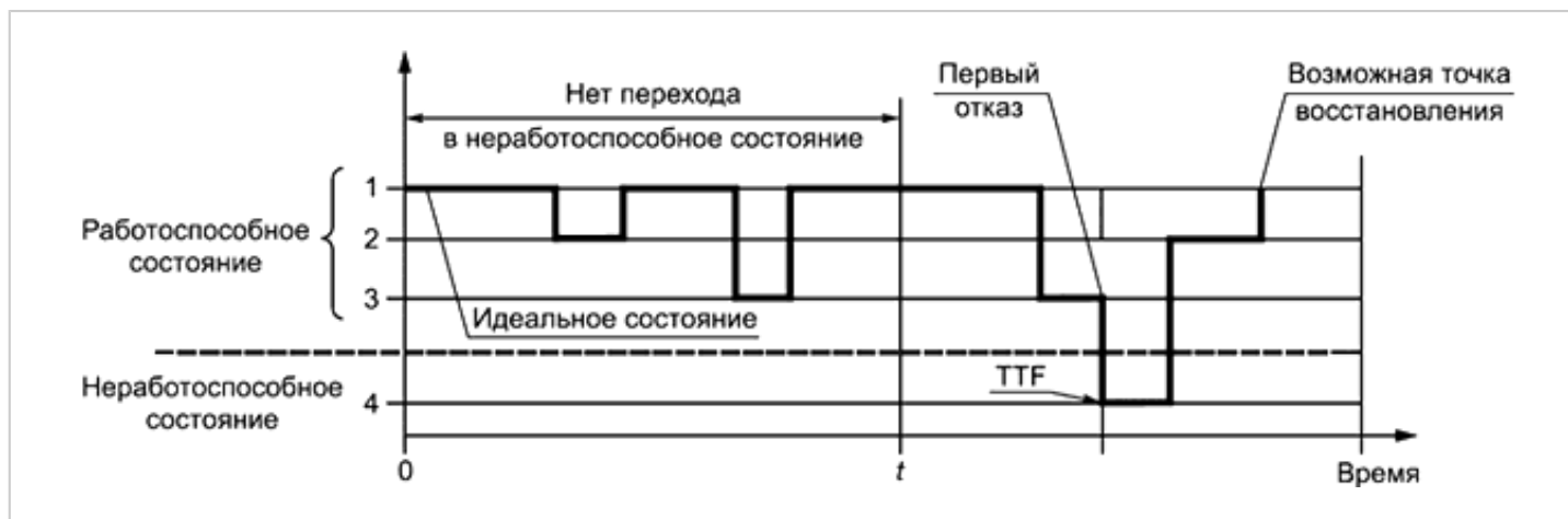
Рисунок 22 - Пример изменения состояний системы за период времени [0, t]
