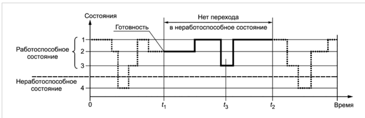
Рисунок 23 - Пример изменения состояний системы в течение периода времени [t_1, t_2]
