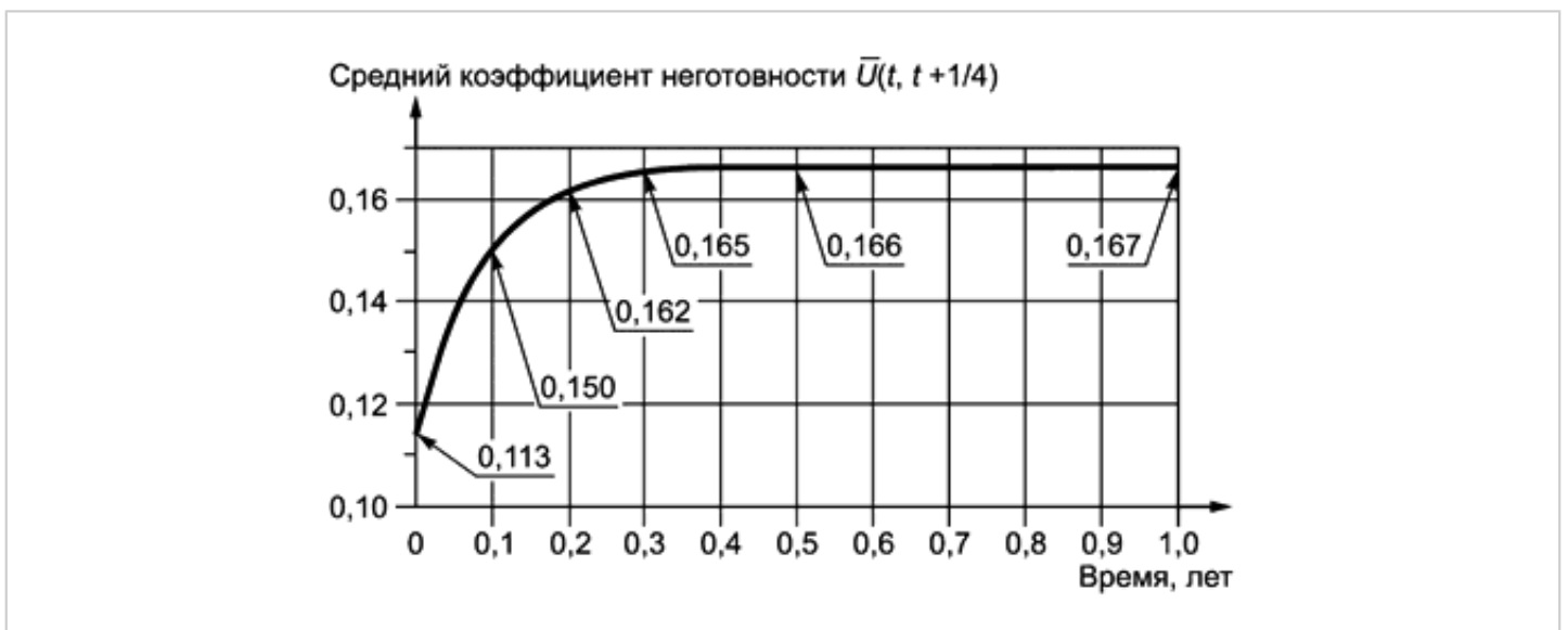
Рисунок 44 - График зависимости от времени среднего коэффициента неготовности \bar{U}(t, t + 1/4)
