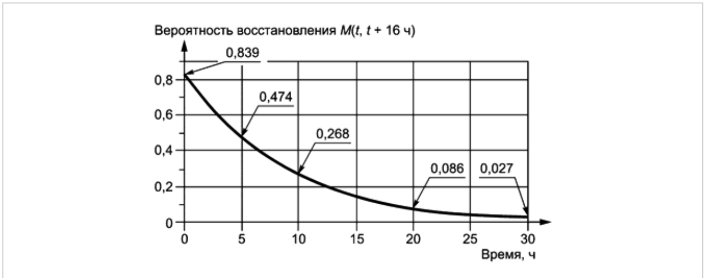
Рисунок 47 - График зависимости от времени M(t, t+16 ч)
