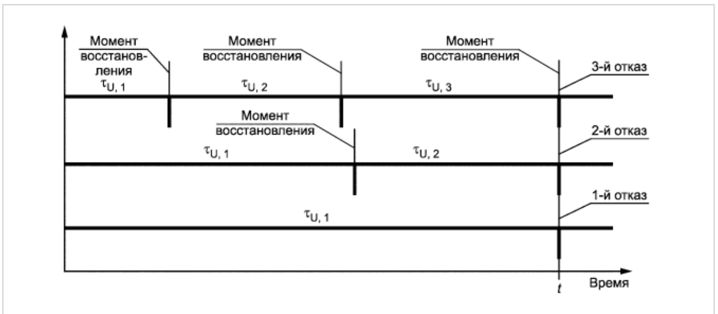
Рисунок 33 - Выборка возможного количества отказов за время восстановления t
