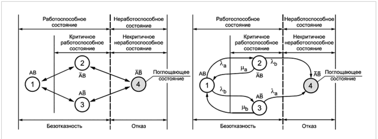
Рисунок 24 - Диаграмма состояний и марковская диаграмма для вычисления вероятности безотказной работы
