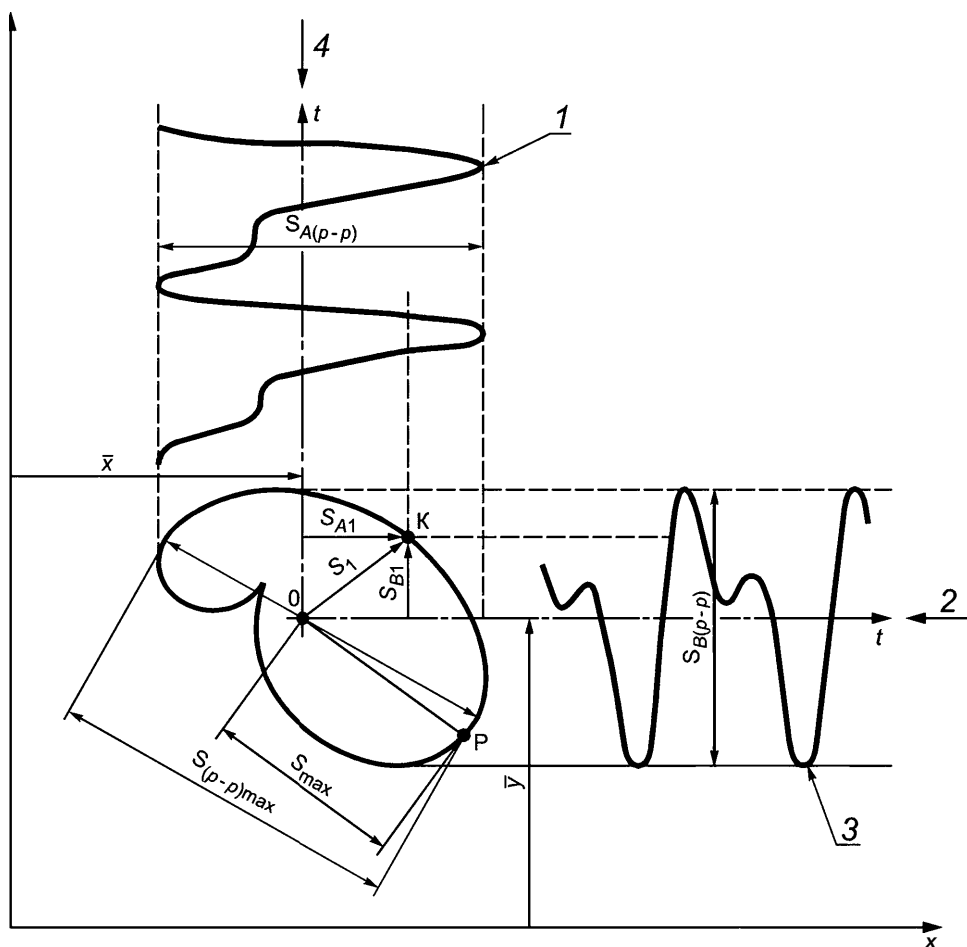
Рисунок А.2 — Траектория движения вала
